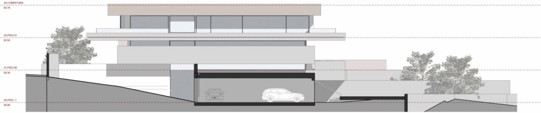
ALÇADO SUL (LOTE 2) 1:100
