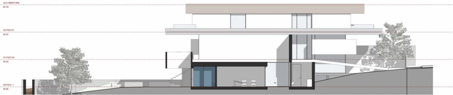
ALÇADO NORTE (LOTE 2) 1:100
