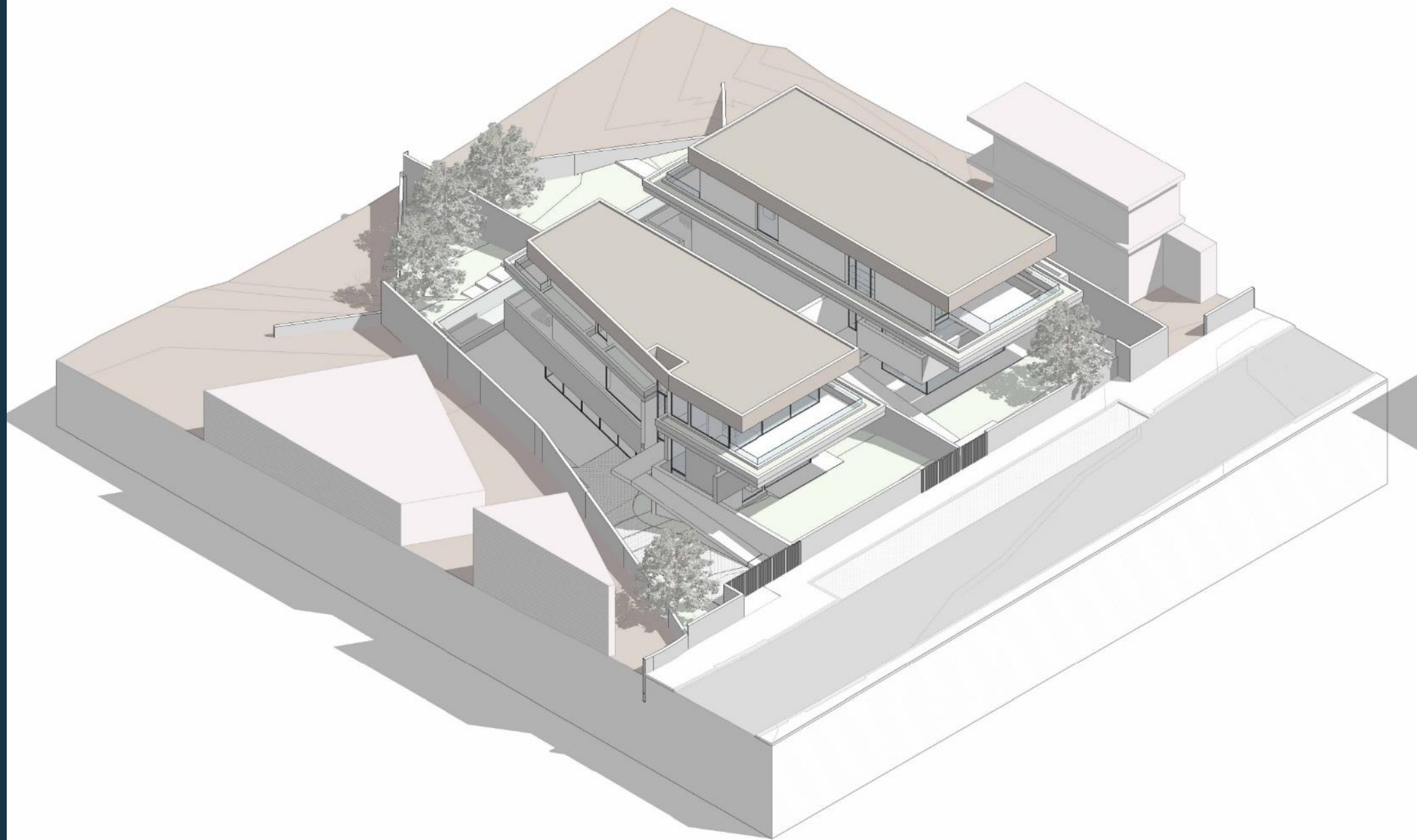
AXONOMETRIA NORTE
