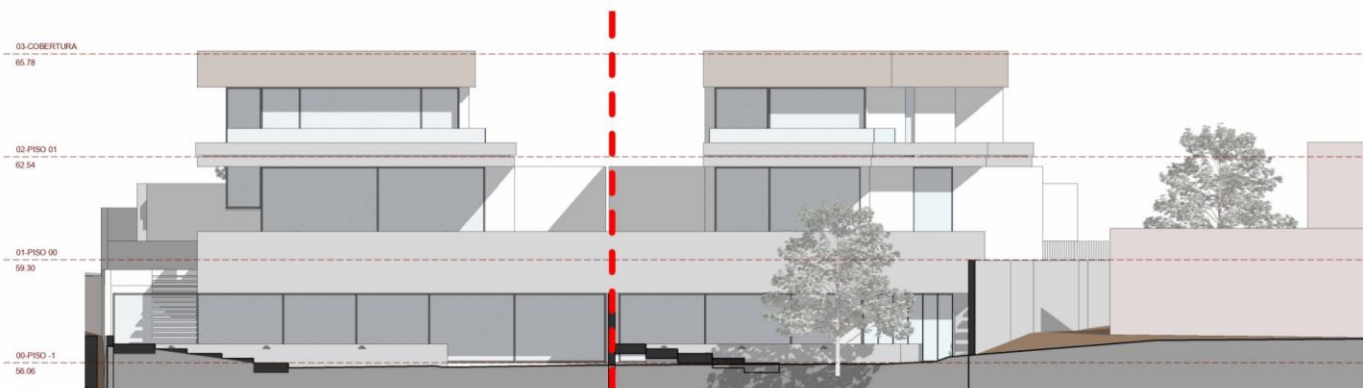
ALÇADO NASCENTE 1:150
