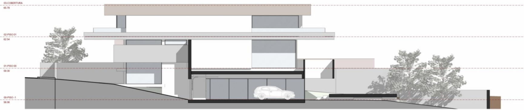
ALÇADO SUL (LOTE 1) 1:100
